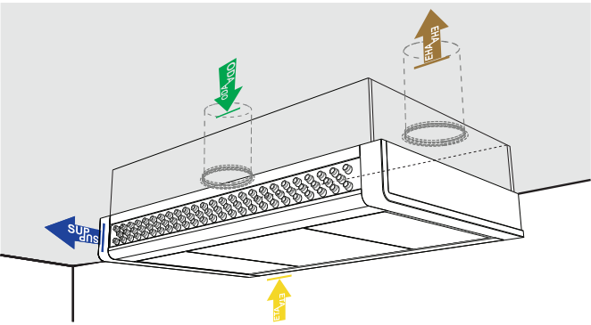
Uitvoering 1 Inbouw met bovenaansluiting
