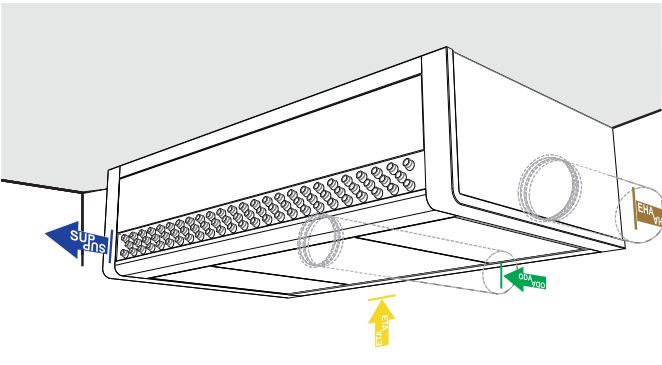
Uitvoering 4 Opbouw met achteraansluiting
