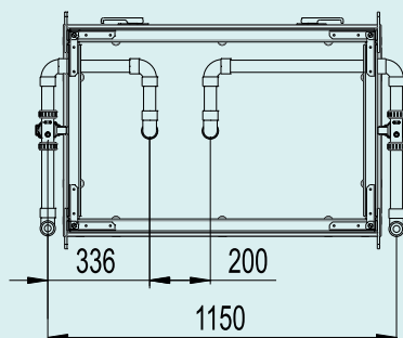
onderaanzicht
