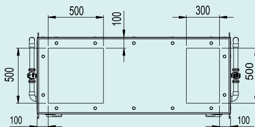
bovenaanzicht met bovenaansluiting
