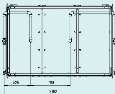
onderaanzicht
