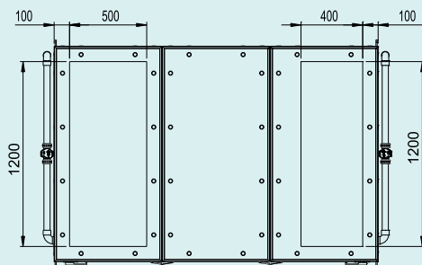
bovenaanzicht met bovenaansluiting
